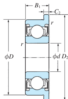
2RS シールド形
