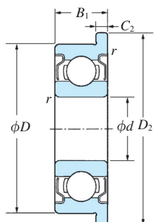
ZZ シールド形
